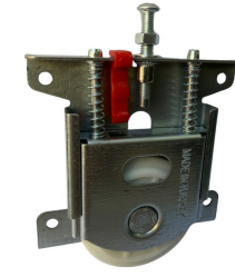
BST-104 PKM 80 SÜRGÜ TEKER BST-104 PKM 80 SLIDING DOOR WHEEL
