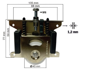
BST-107 SÜRGÜ TEKER PREMIUM BST-107 PKM 100 SLIDING DOOR WHEEL
