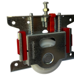
BST-106 PKM 100 SÜRGÜ TEKER BST-106 PKM 100 SLIDING DOOR WHEEL
